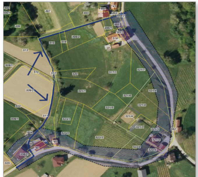
Odsek vodovoda, predviden za izvedbo v letu 2020
